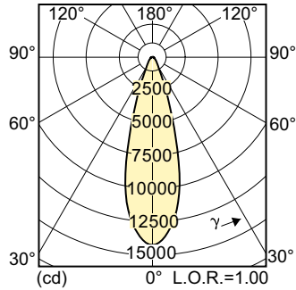
CDM-R Elite 70W /942 PAR30L 30D
