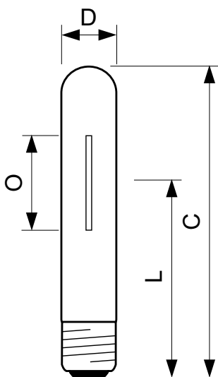
SON-T, E27/E40
