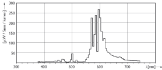
MST SON- T PIA Plus Plus 50W/70W E27
