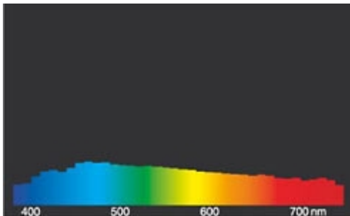
Lichtfarbe 840 Spectralux® weiß (21)
