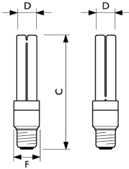
MASTER PL-E E27
