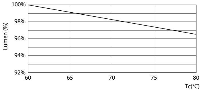
LEDtube_PLCT_8W_30K_LumenVsTc-LMP
