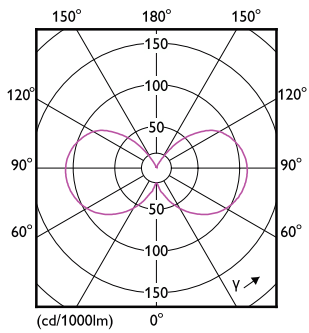
LEDClassic LATAM B11 4,5W E27 850 CL-LDD
