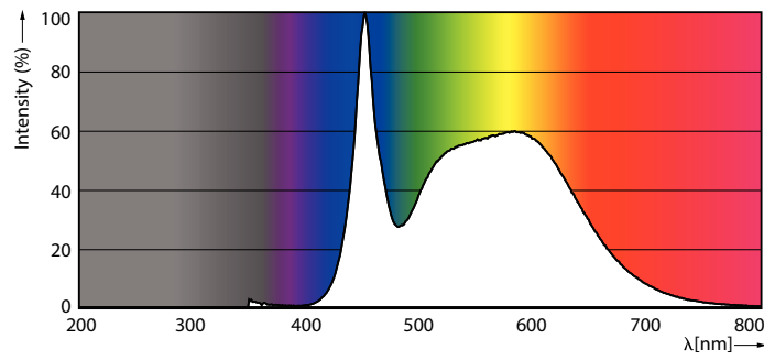
LEDClassic LATAM 4,5W B11 E27 850 CL-POC
