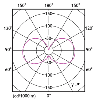
LEDcandle MAS SLR B35 2,5W E14 927 CL-LDD
