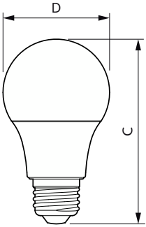
5.5A19/LED/950/FR/P/E26/ND 4/2CT
