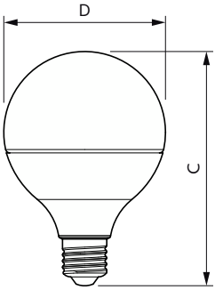
LEDGlobe13-175W G95 E27 CDL100-240V BR
