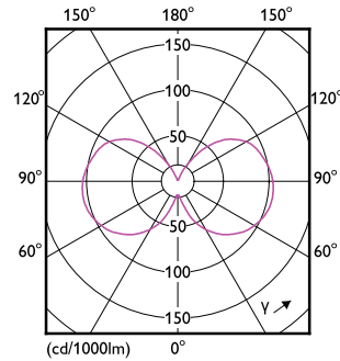
LEDbulb CLA G16,5 4,5W E27 827 CL
