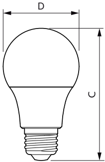
6A19/LED/850/FR/P/ND 4/2FB
