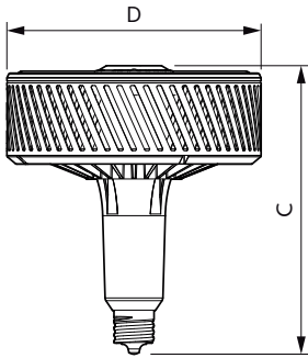
TrueForce HB 140W E40 840 NB LA
