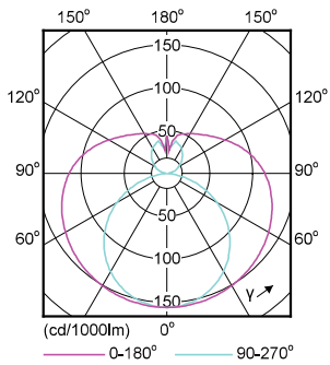
LEDTube_LEDtube 600mm 8-18W 800lm 4000K G13
