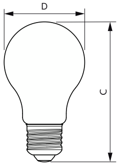
LEDClassic 48W A60 E27 825 100-240V NDLA
