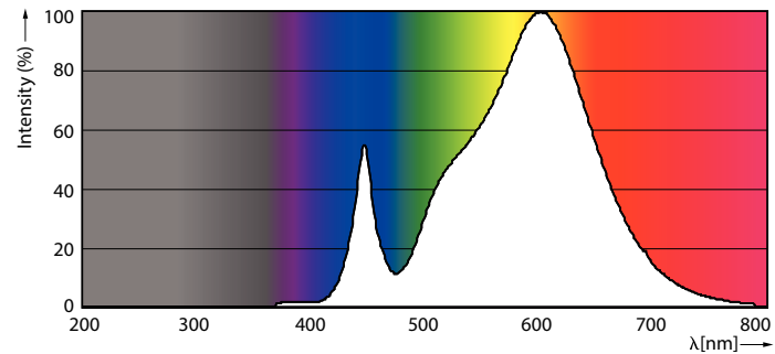
LEDSpot 33W E26 PAR38
