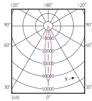
LEDspot E27 PAR30L 35W 6000K
