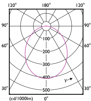
LEDspots RCA 5,5W PAR16 GU10 827 120D-LDD
