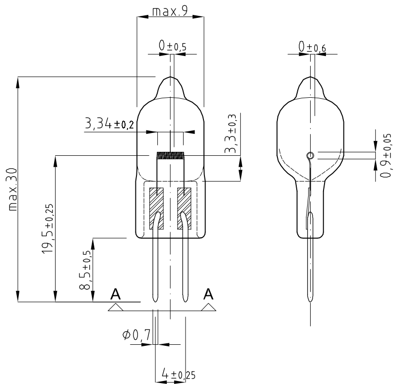
Schnitt A-A
