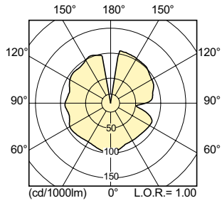
CDO-TT Plus 70W /828 E27
