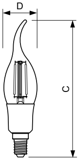
filament 4.5W-40W 470lm NAD 2700K E14D
